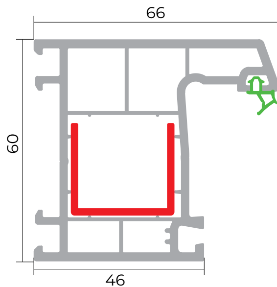
Çərçivə profili
