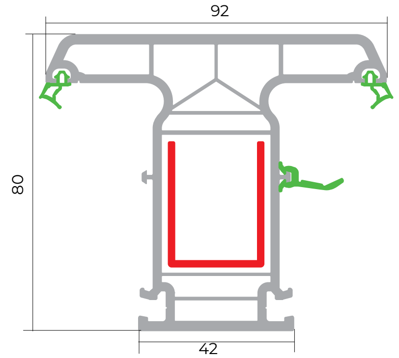
Dirək profili
