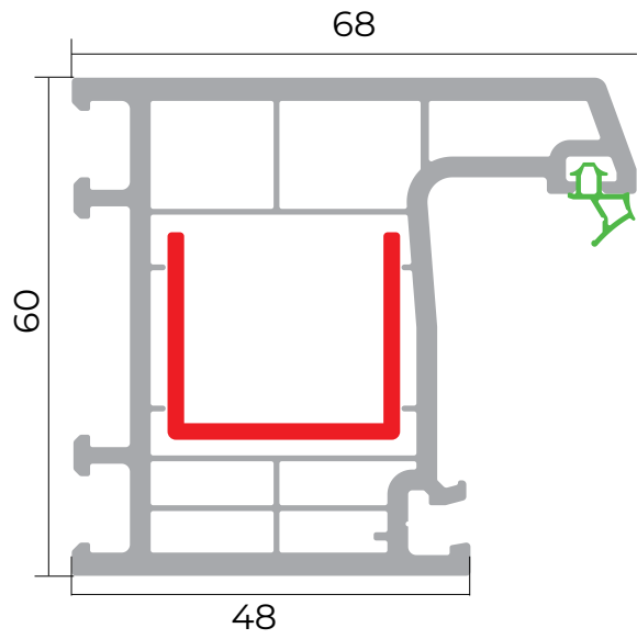
Çərçivə profili
