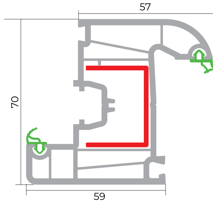
Qanad profili
