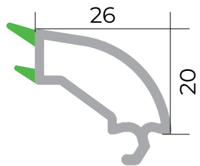
Cüt şüşə ştapiki
