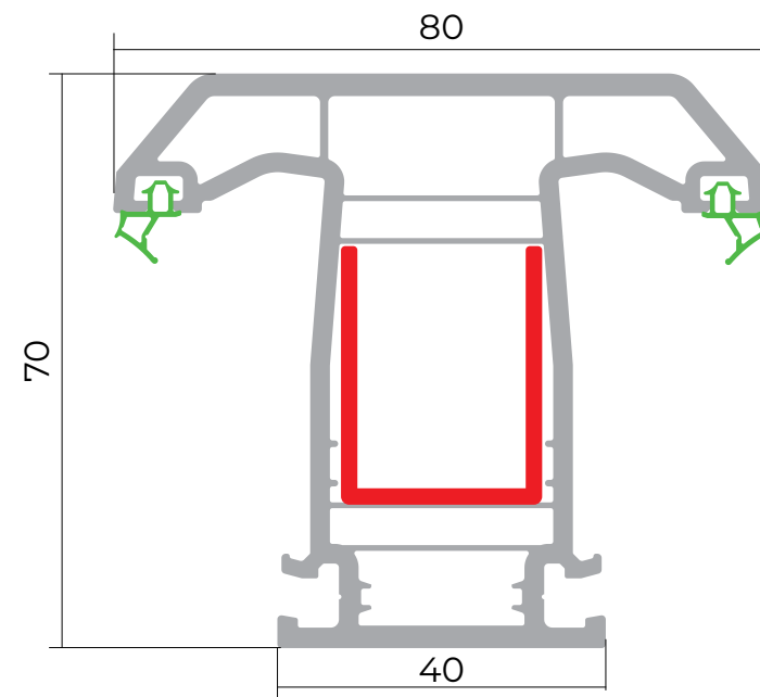
Dirək profili
