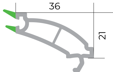
Tək şüşə ştapiki
