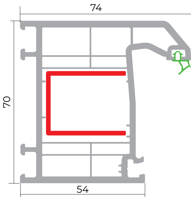
Çərçivə profili
