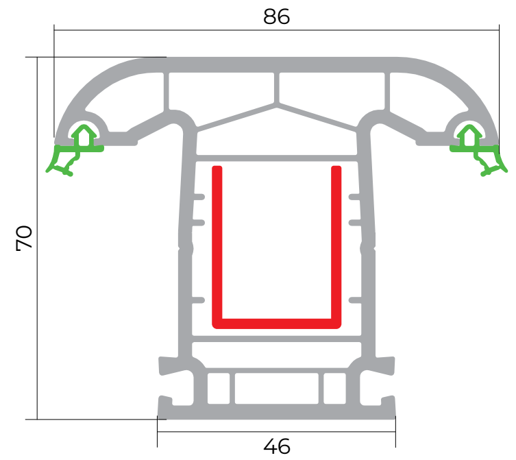
Dirək profili
