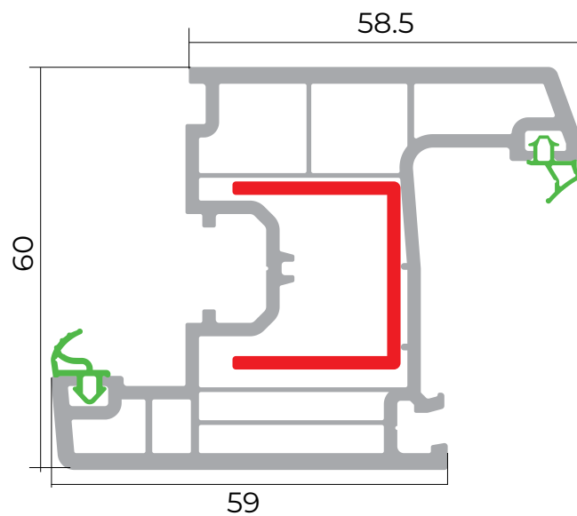
Qanad profili
