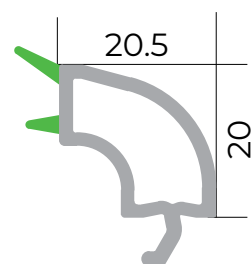
Cüt şüşə ştapiki
