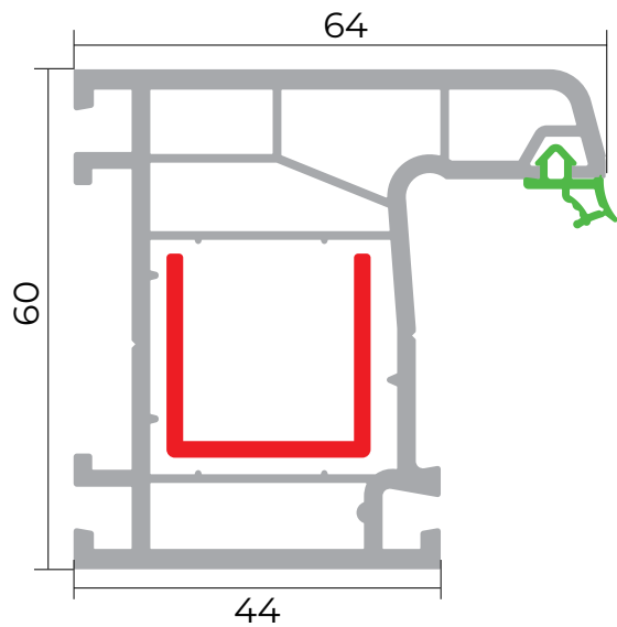
Çərçivə profili
