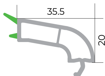
Tək şüşə ştapiki
