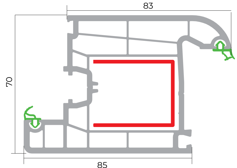
Qapı qanad profili
