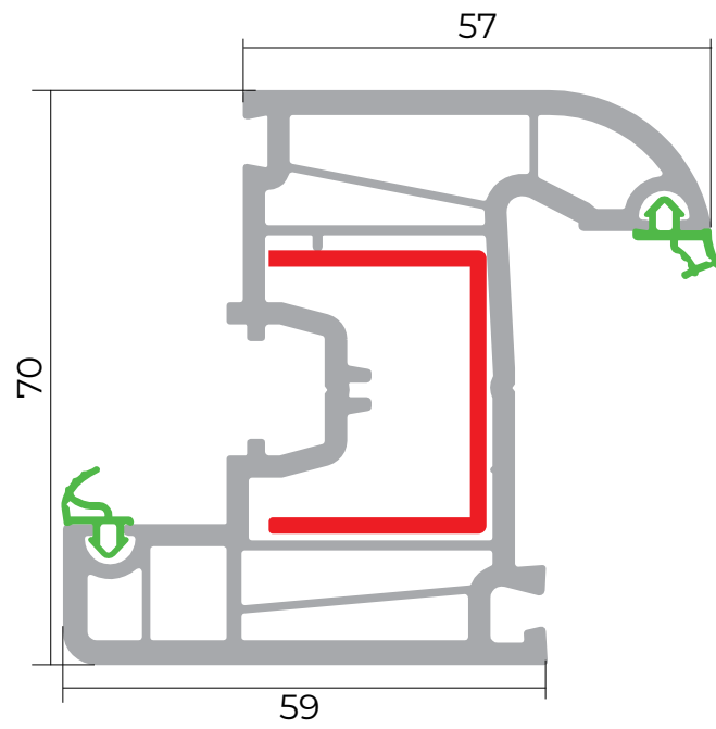
Düz qanad profili
