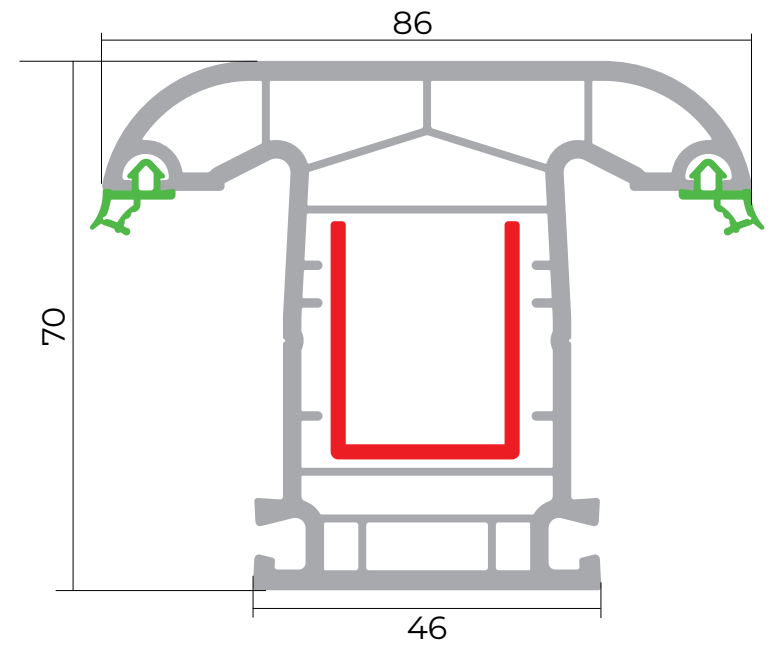
Dirək profili
