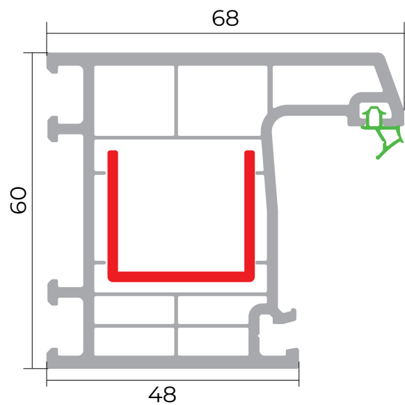
Çərçivə profili
