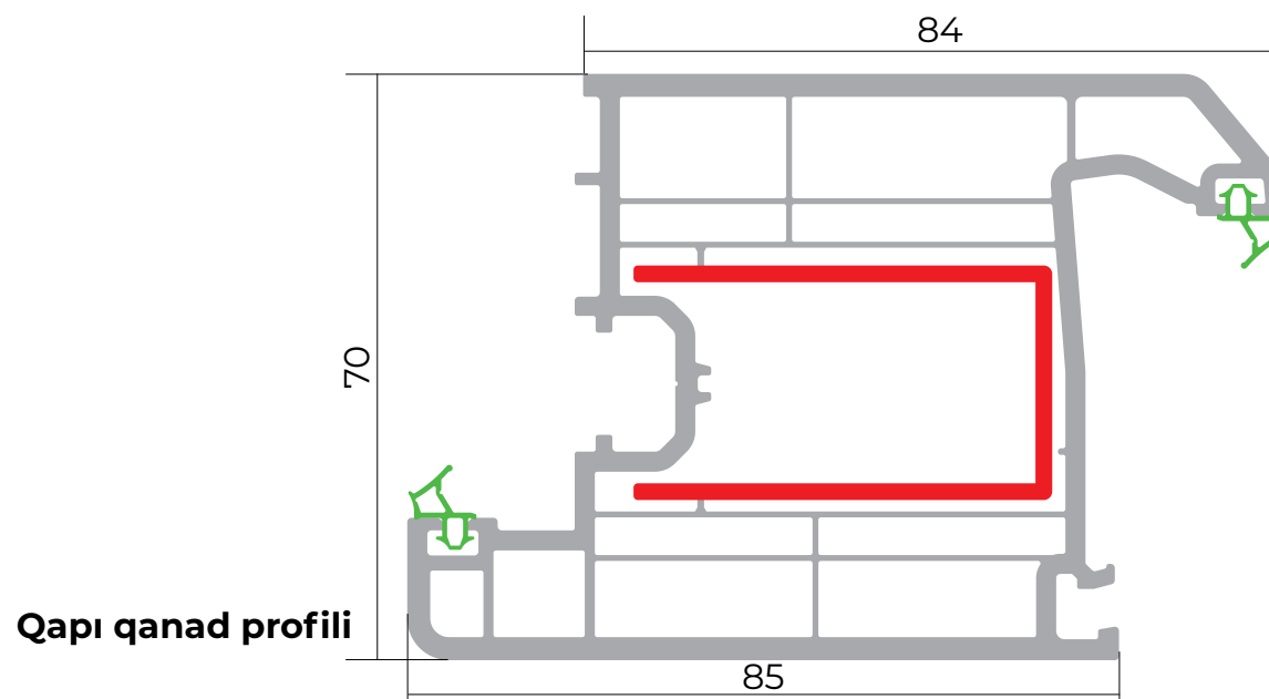
Qanad profili
