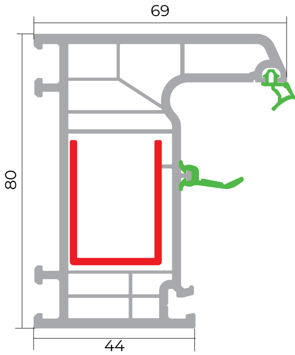
Çərçivə profili
