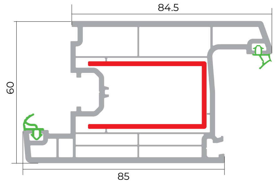
Qapı qanad profili
