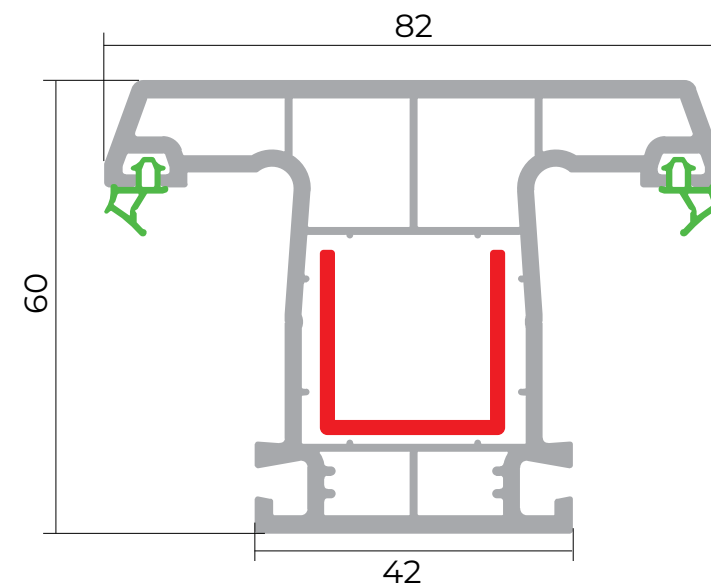
Dirək profili
