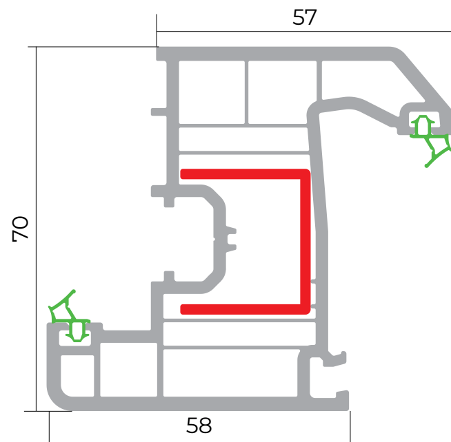
Qanad profili
