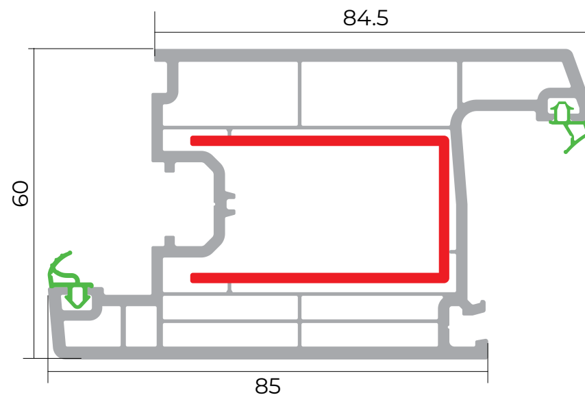
Qapı qanad profili
