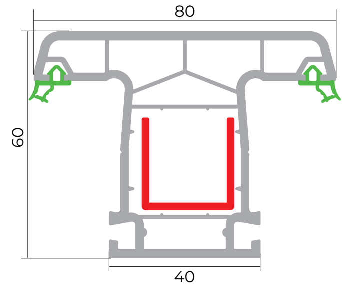
Dirək profili
