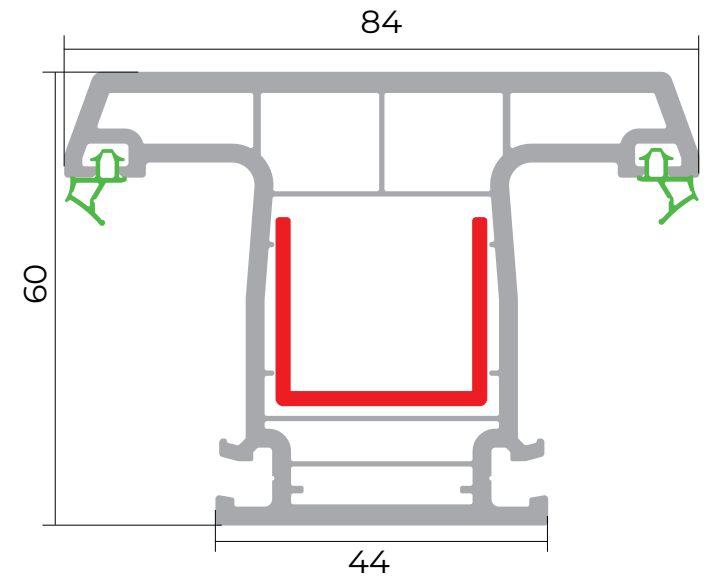
Dirək profili
