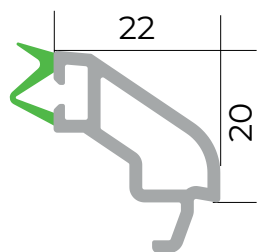
Cüt şüşə ştapiki
