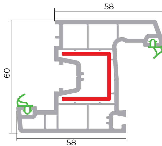
Qanad profili
