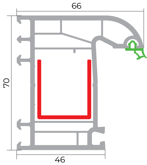
Çərçivə profili
