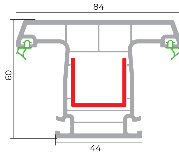
Dirək profili
