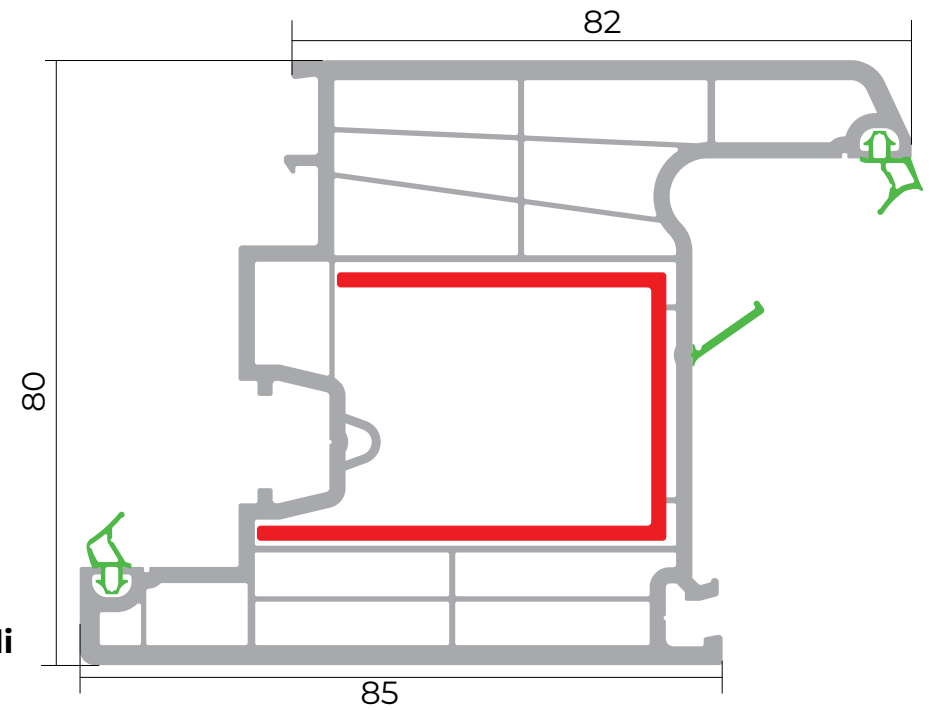
Dirək profili
