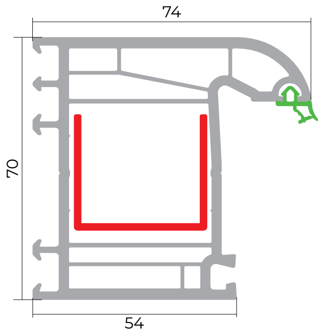
Çərçivə profili
