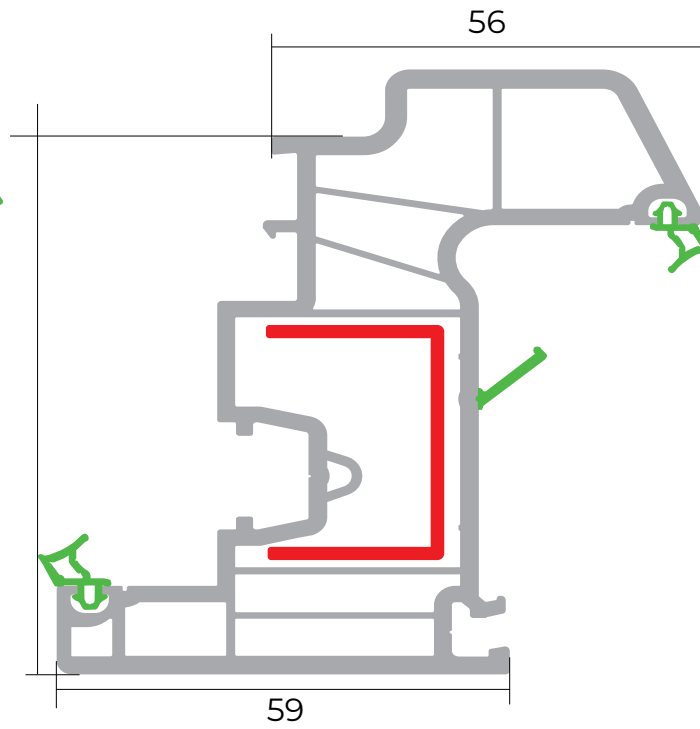
Qanad profili
