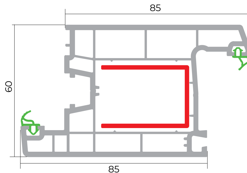
Qapı qanad profili
