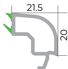
Cüt şüşə ştapiki
