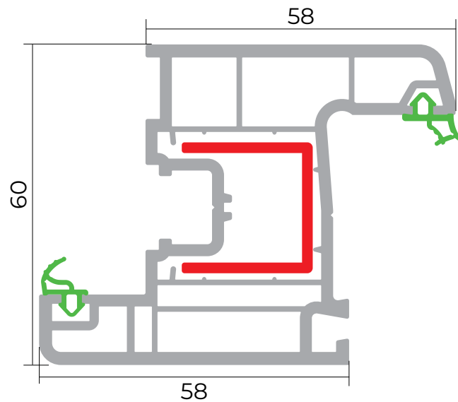
Qanad profili
