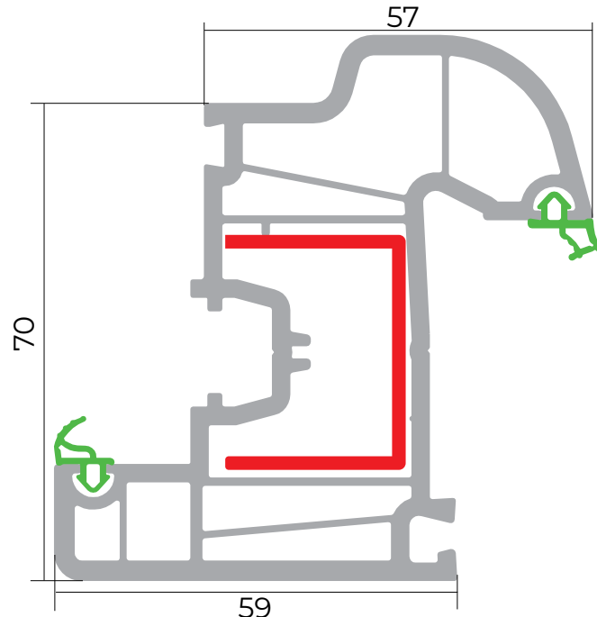
Dekorativ qanad profili
