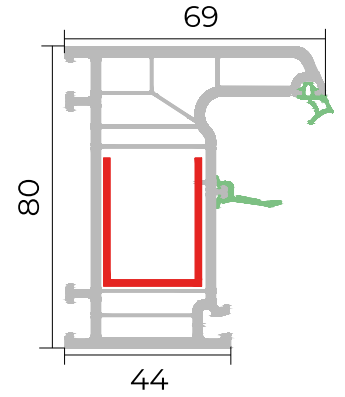
Çərçivə profili Frame profile
