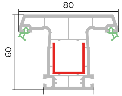
Dirək profili Mullion profile
