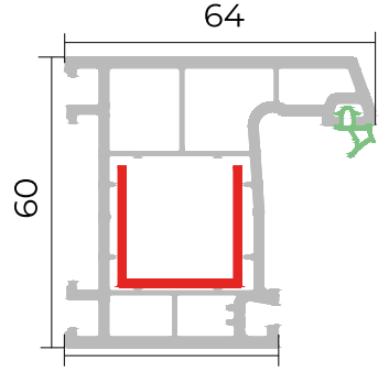
Çərçivə profili Frame profile
