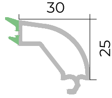
Cüt şüşə ştapiki Double glazing bead
