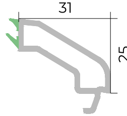
Üçlü şüşə ştapiki Triple glazing bead
