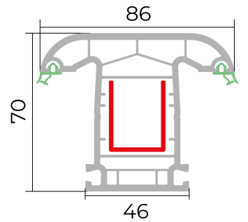
Dirək profili Mullion profile
