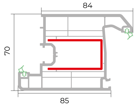
Qapı qanad profili Door sash profile
