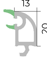
Üçlü şüşə ştapiki Triple glazing bead
