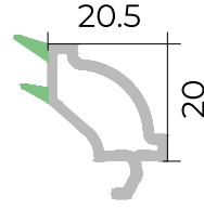
Dekorativ cüt şüşə ştapiki Decorative double glazing bead
