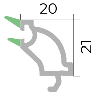
Cüt şüşə ştapiki Double glazing bead
