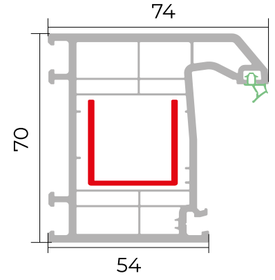
Çərçivə profili Frame profile
