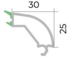
Cüt şüşə ştapiki Double glazing bead
