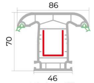
Dirək profili Mullion profile
