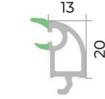
Üçlü şüşə ştapiki Triple glazing bead
