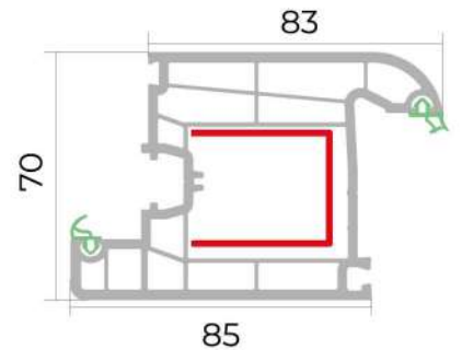
Qapı qanad profili Door sash profile
