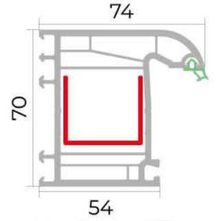
Çərçivə profili Frame profile
